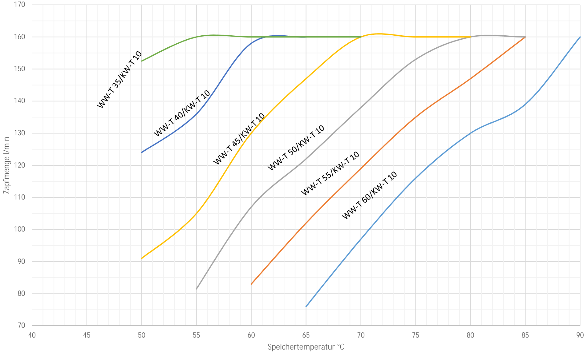
Auslegungsdiagramm 4er Kaskade
