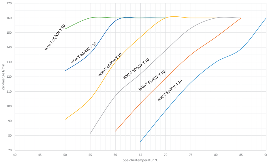
Auslegungdiagramm FWS40 HYDRO
